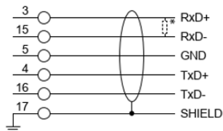
RS-422 原理线路图
