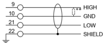
CAN 原理线路图
