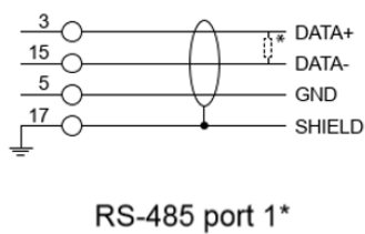
RS-485 原理线路图
