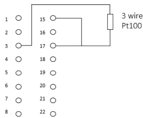
三线制 Pt100 原理线路图:
