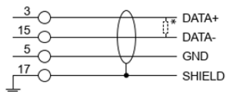
RS-485 原理线路图
